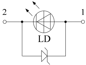
Zener Diode
